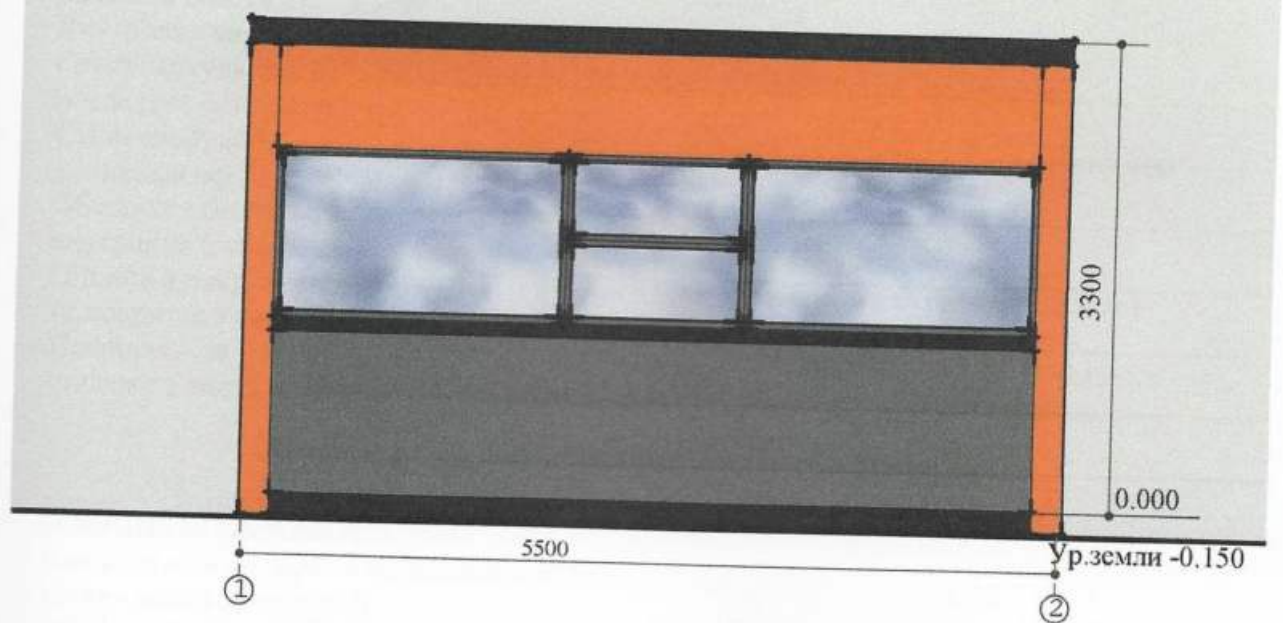
Боковий фасад
