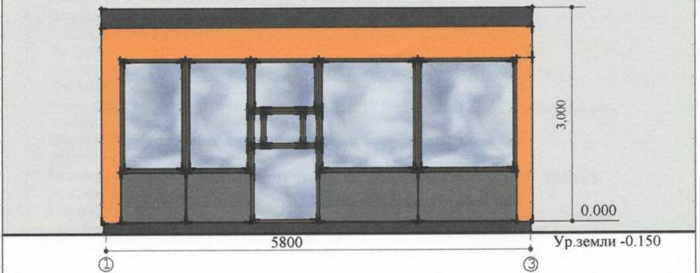
Боковий фасад
