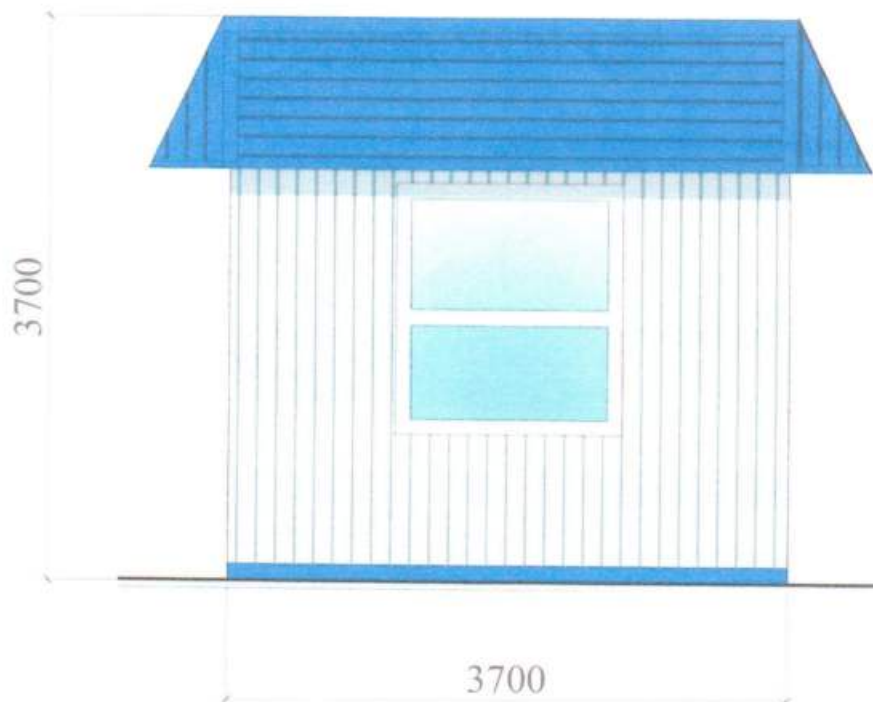
Головний фасад ТС М 1:50
