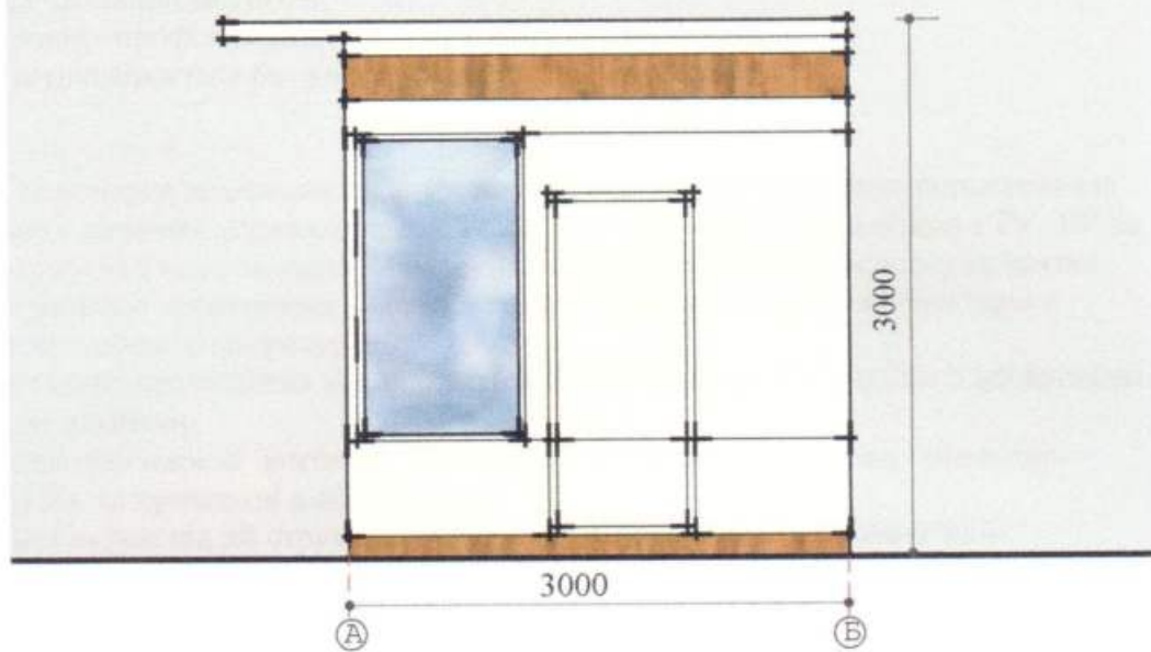
Боковий фасад
