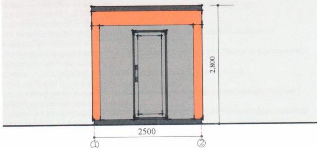
Боковий фасад
