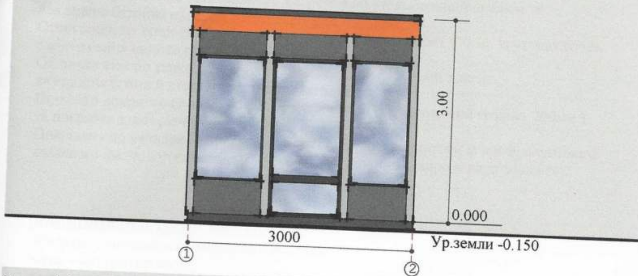
Боковий фасад
