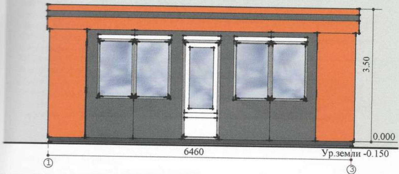
Боковий фасад
