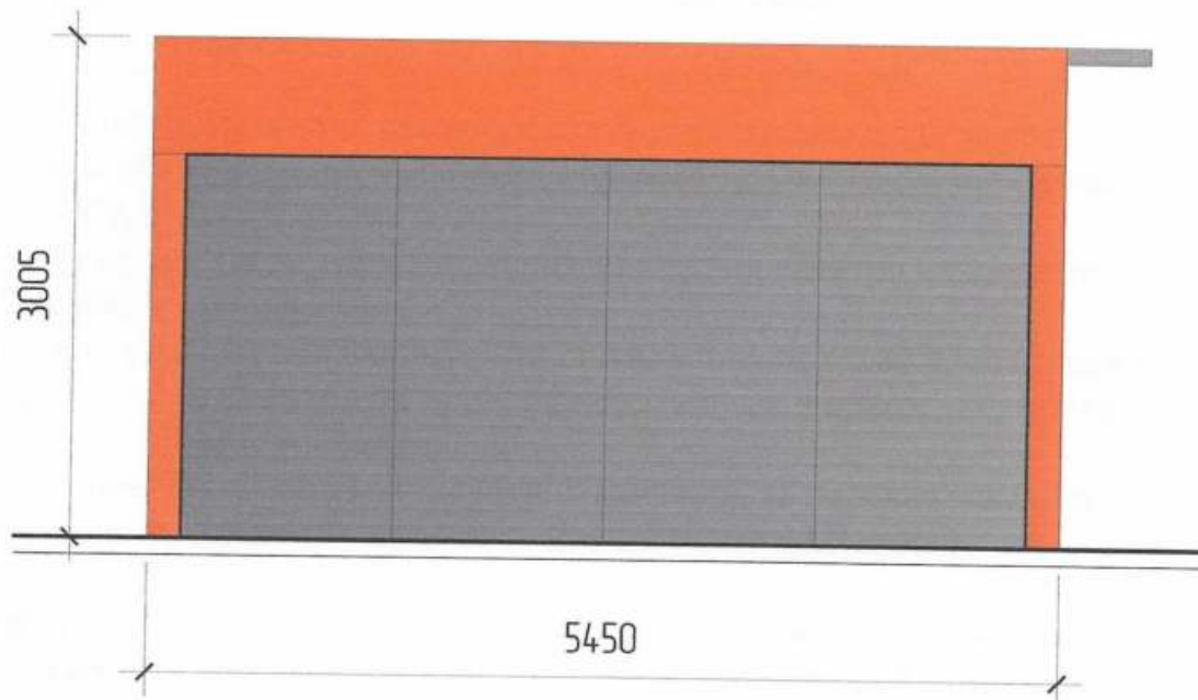
Бічний фасад групи ТС М 1:50
