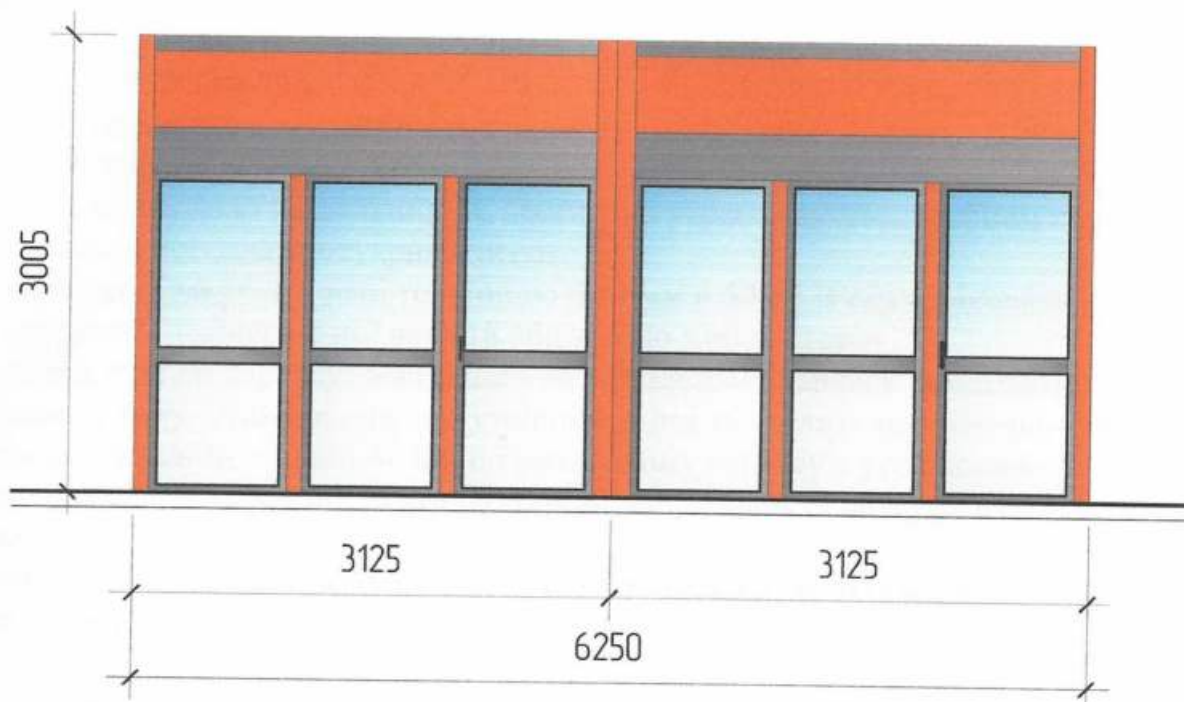
Бічний фасад групи ТС М 1:50
