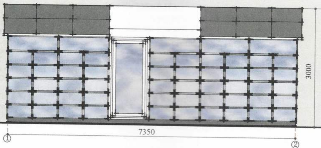
Боковий фасад
