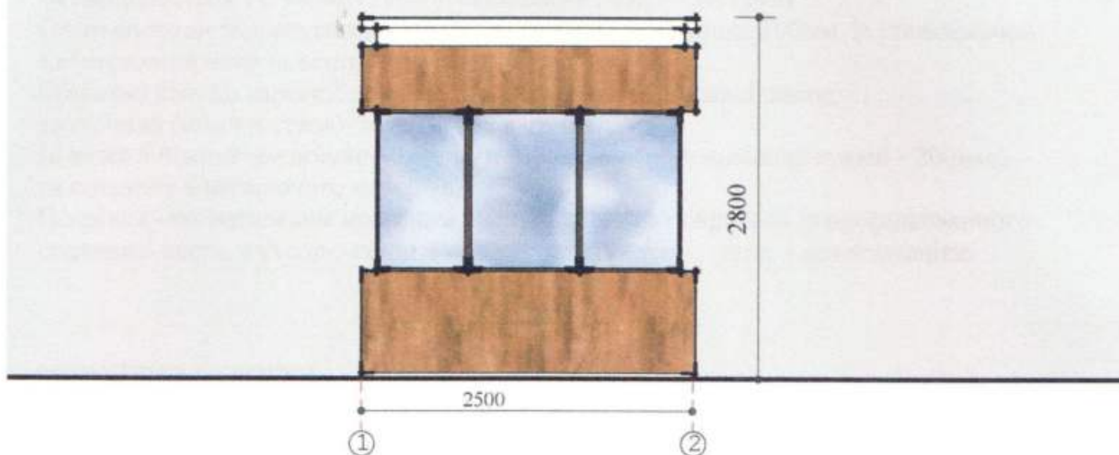
Боковий фасад
