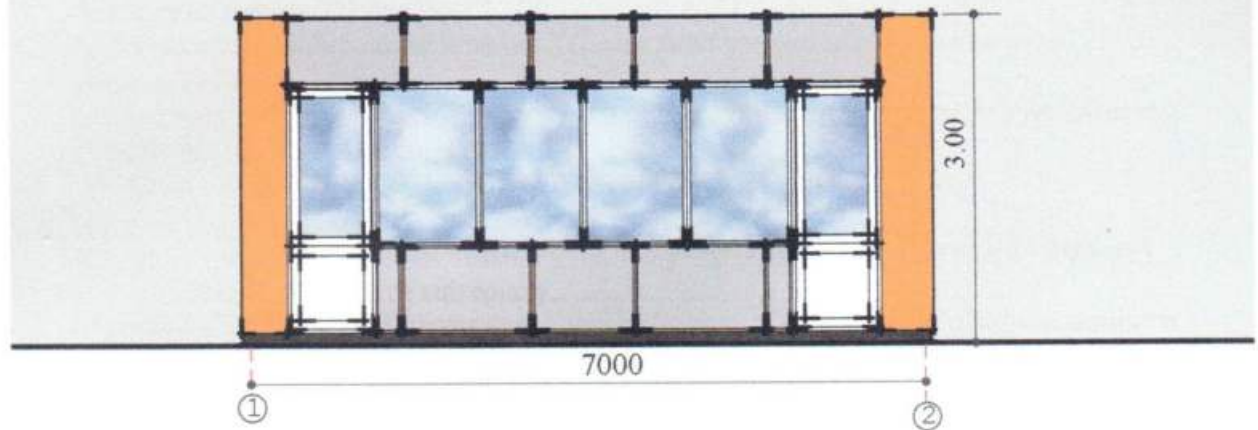
Боковий фасад
