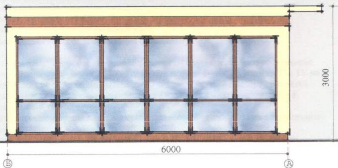
Боковий фасад
