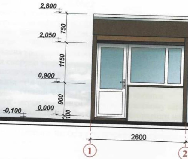
Бічний фасад
