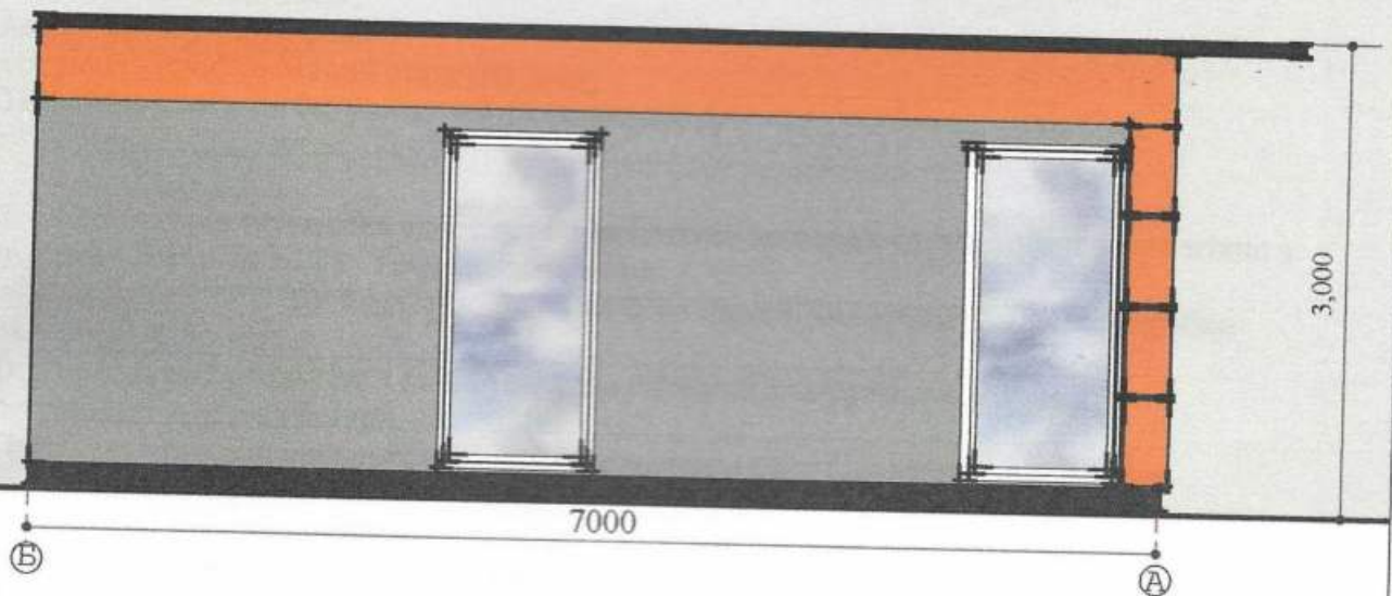
Боковий фасад
