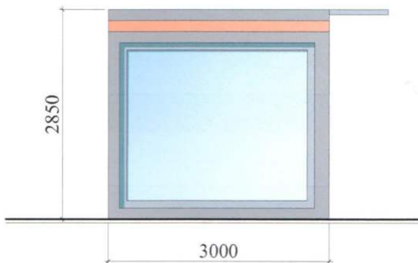
Бічний фасад М 1:50
