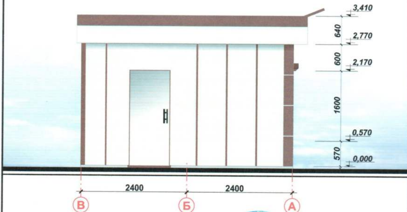
Бічний фасад
