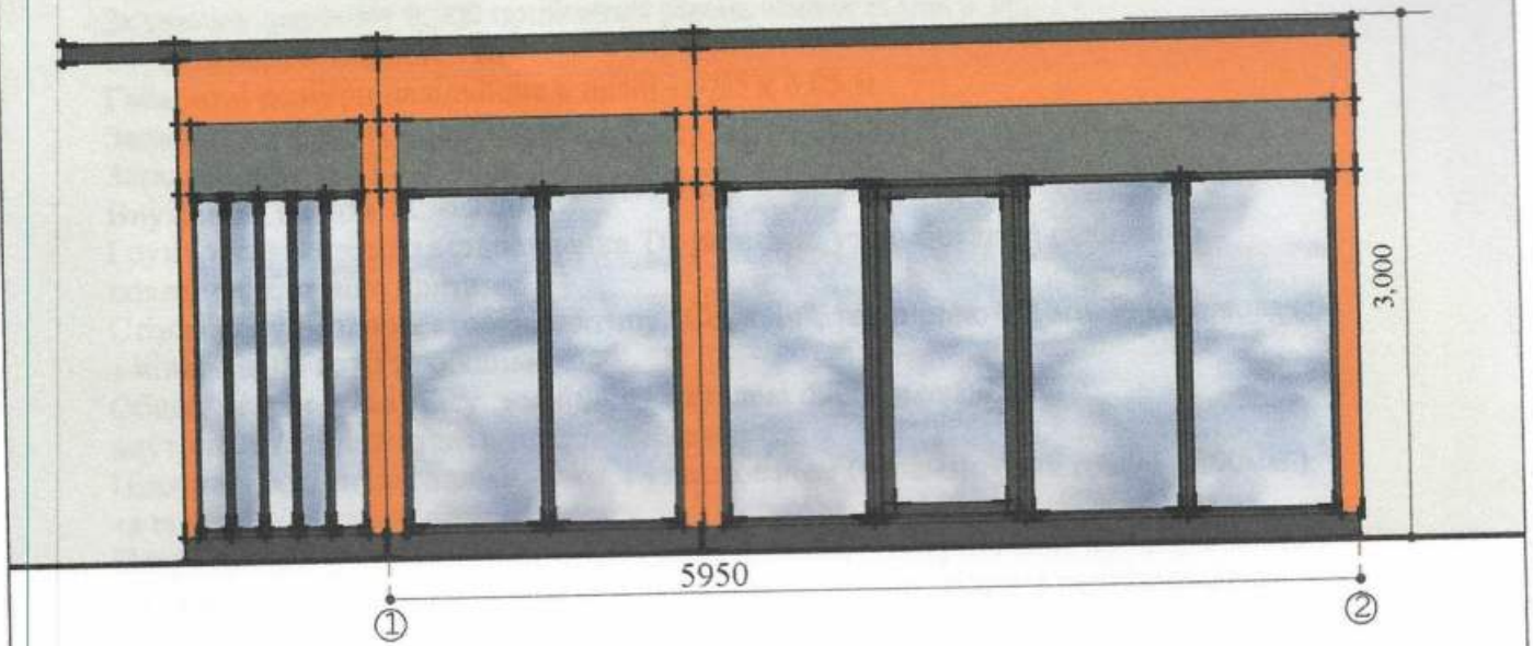
Головний фасад
