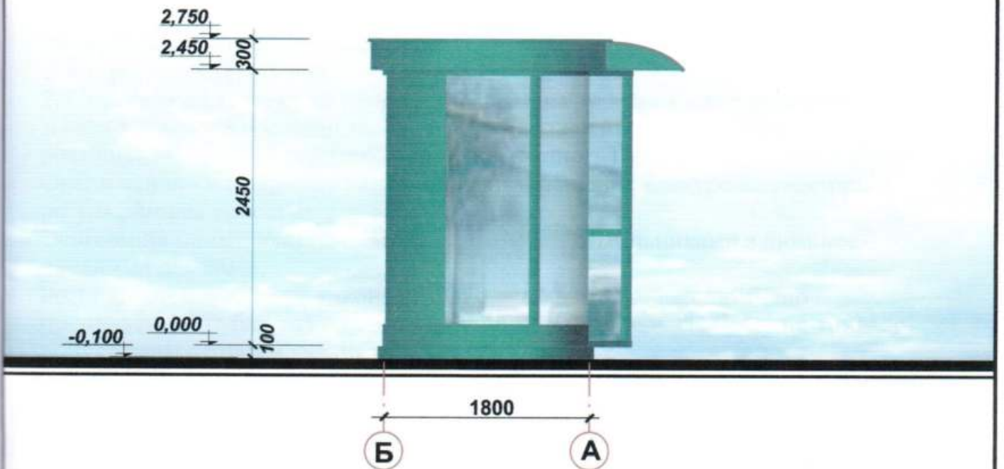
Бічний фасад
