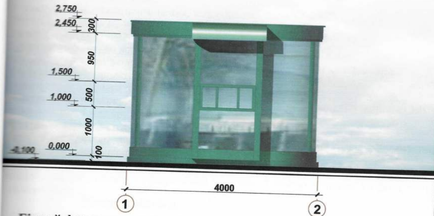
Бічний фасад
