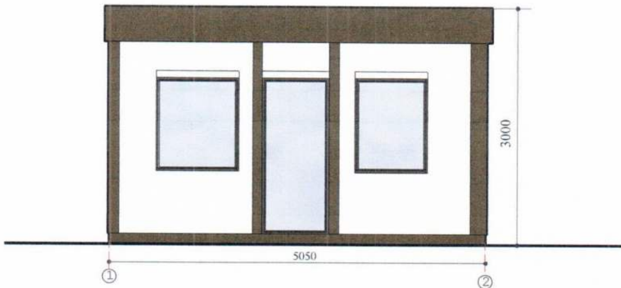
Боковий фасад
