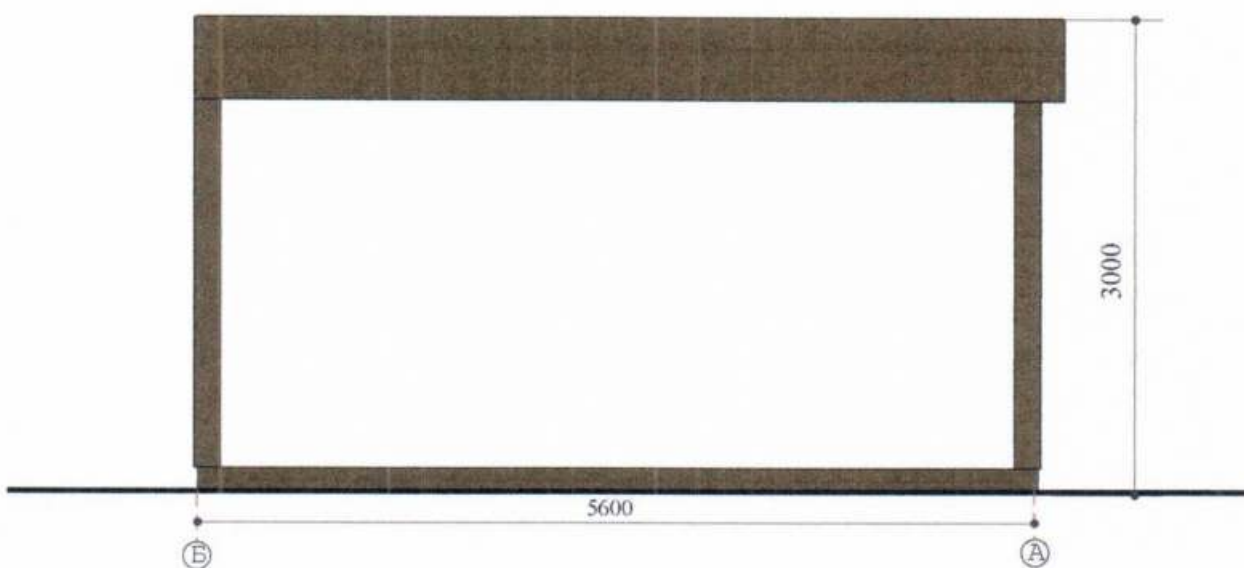
Боковий фасад
