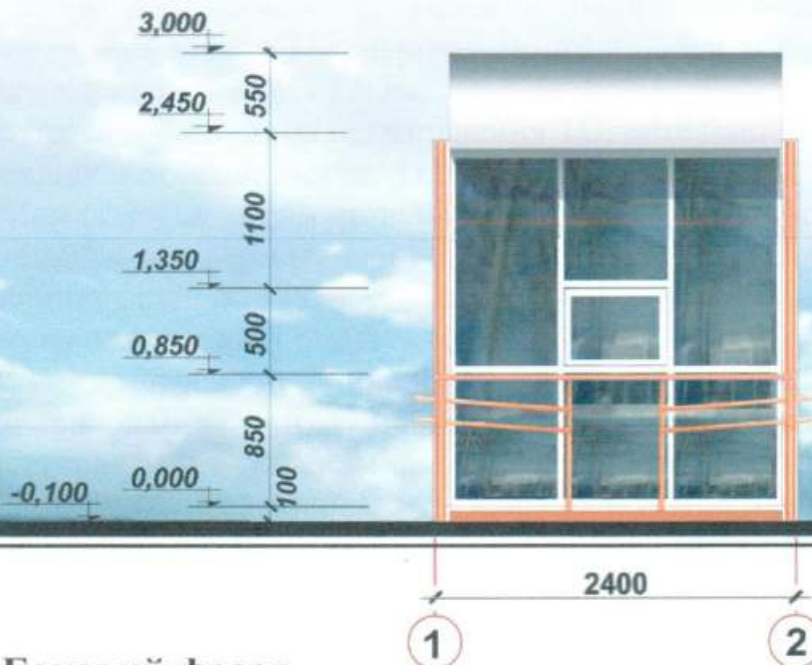
Боковий фасад
