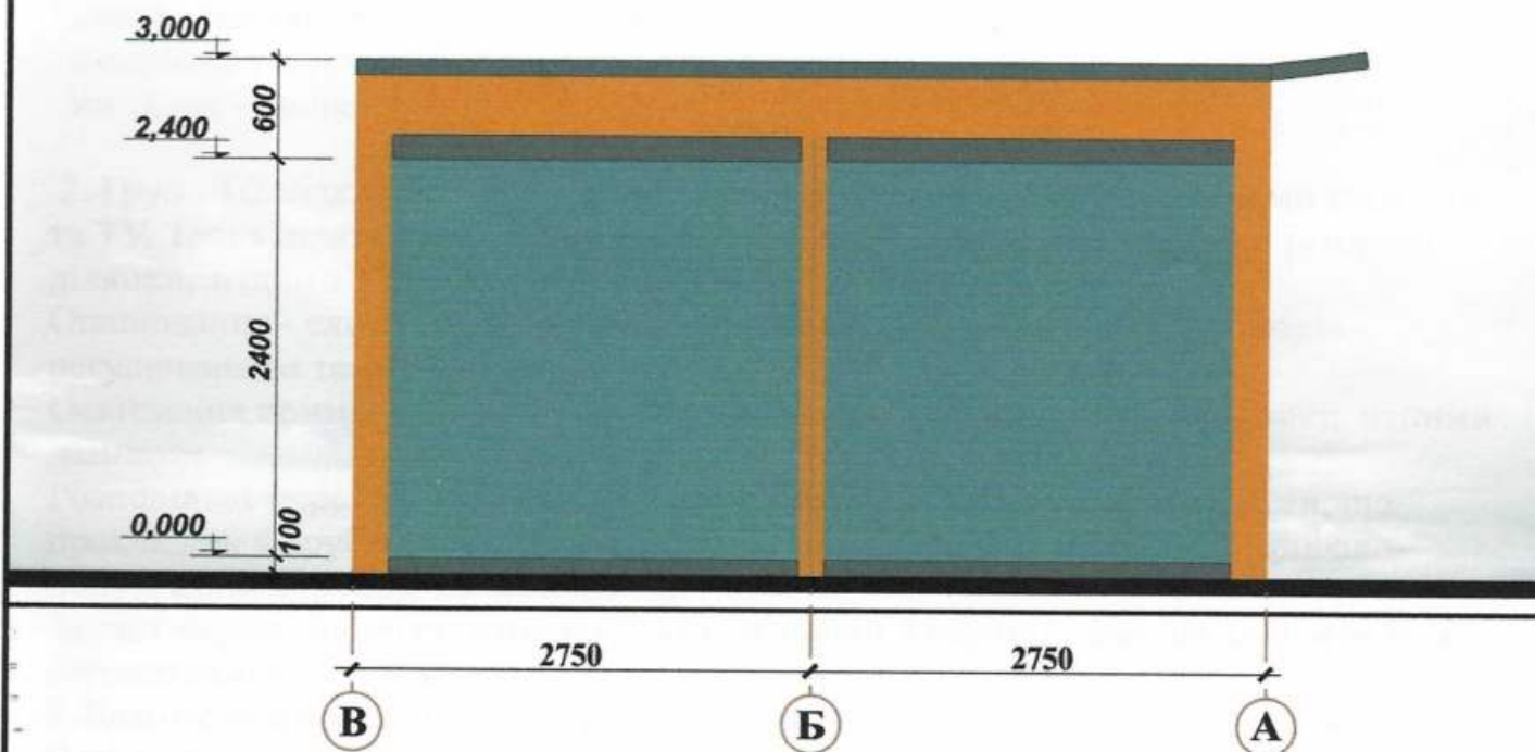
Бічний фасад
