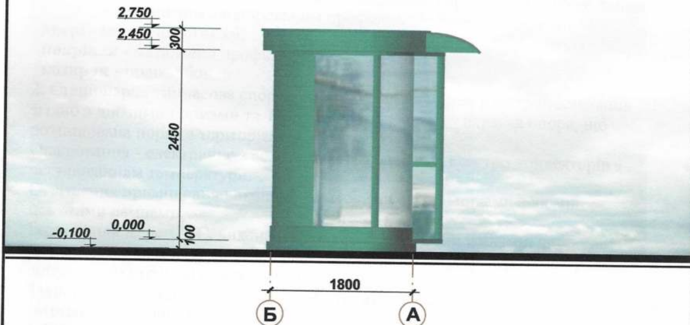
Бічний фасад
