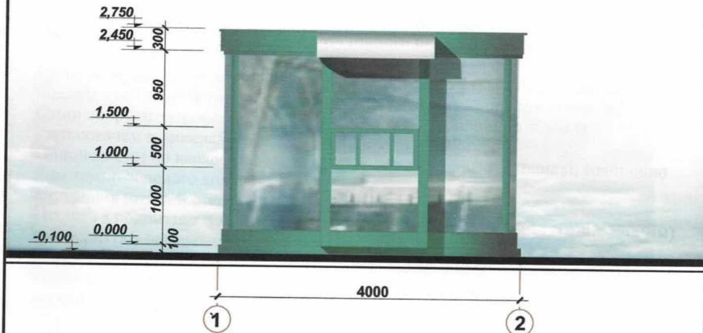
Бічний фасад
