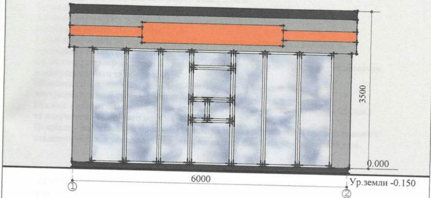
Боковий фасад
