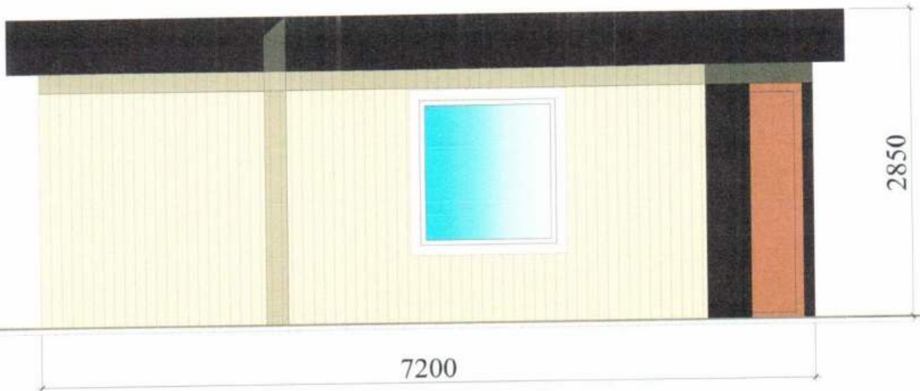
Головний фасад ТС М 1:50
