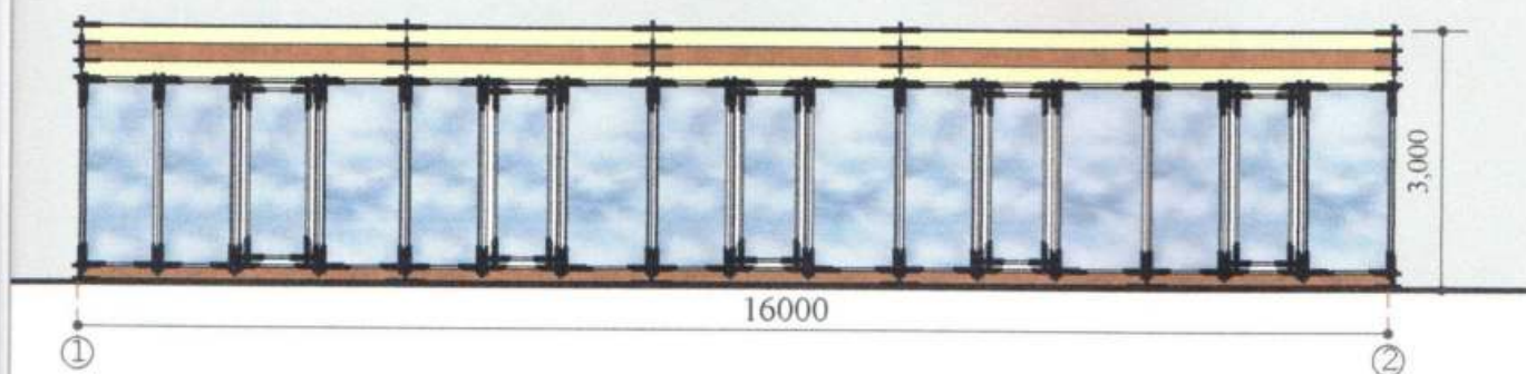
Боковий фасад
