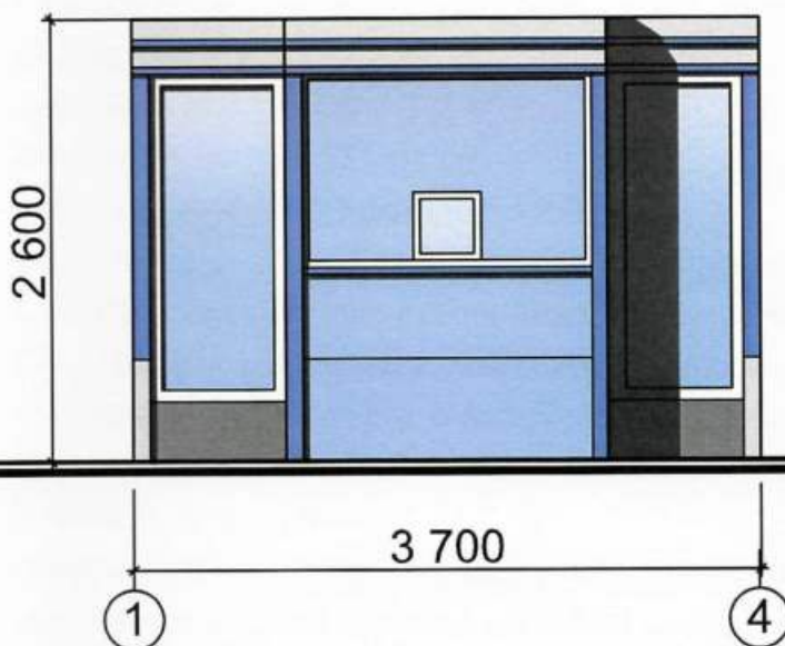
Головний фасад
