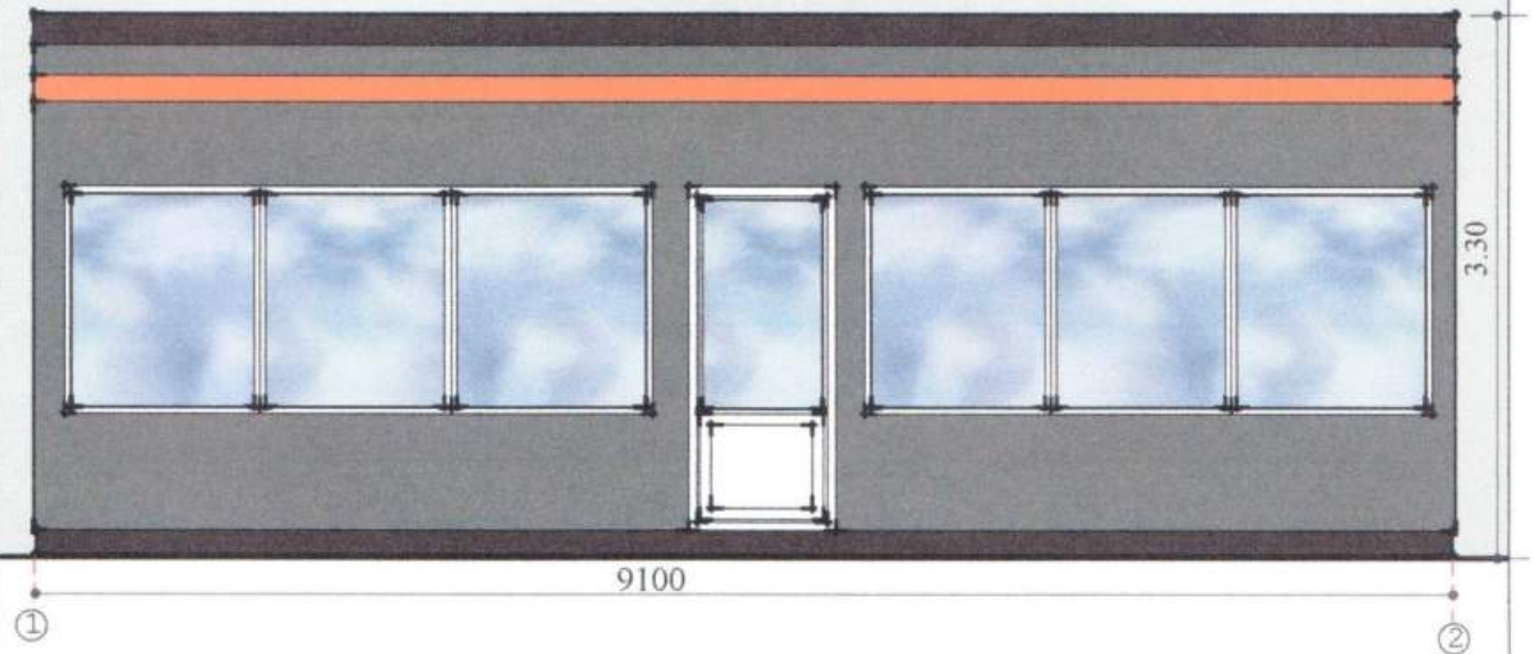
Боковий фасад
