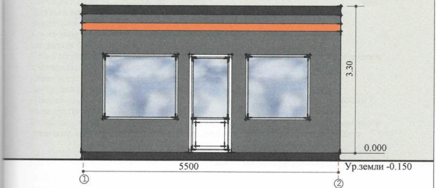
Боковий фасад
