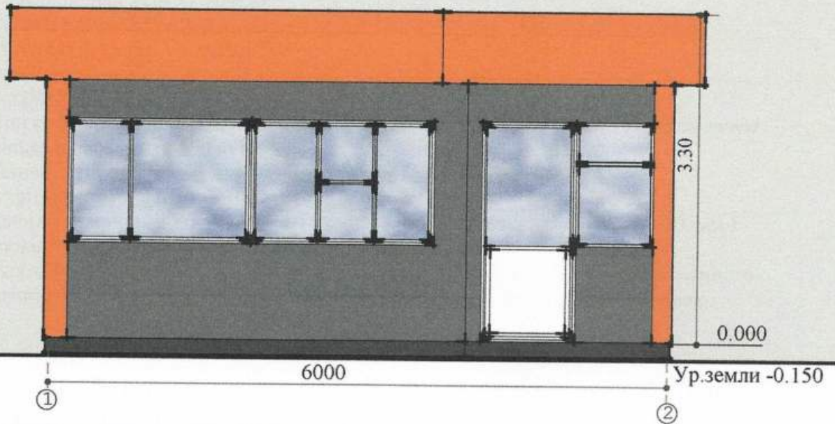
Боковий фасад
