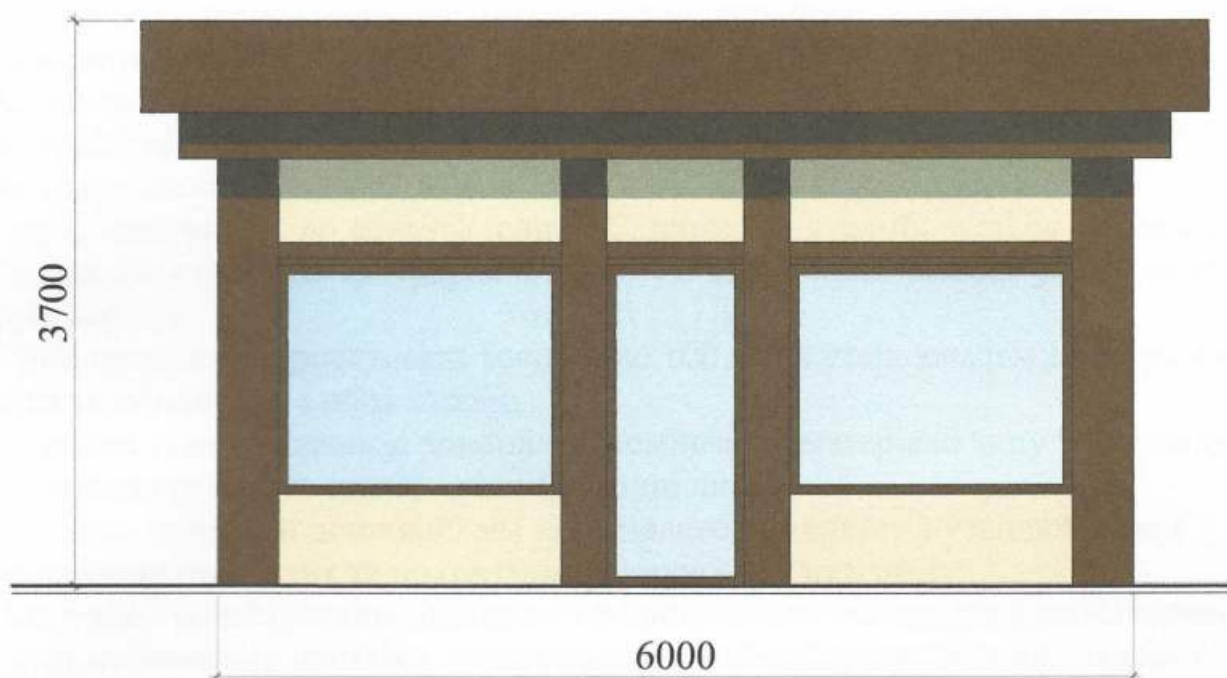
Головний фасад ТС М 1:50
