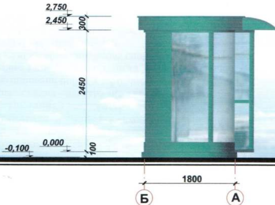
Бічний фасад
