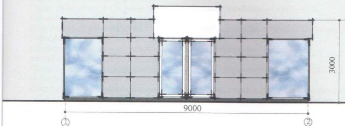
Боковий фасад
