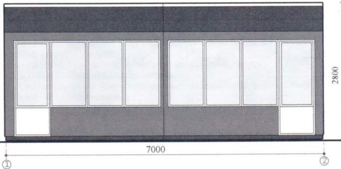
Боковий фасад
