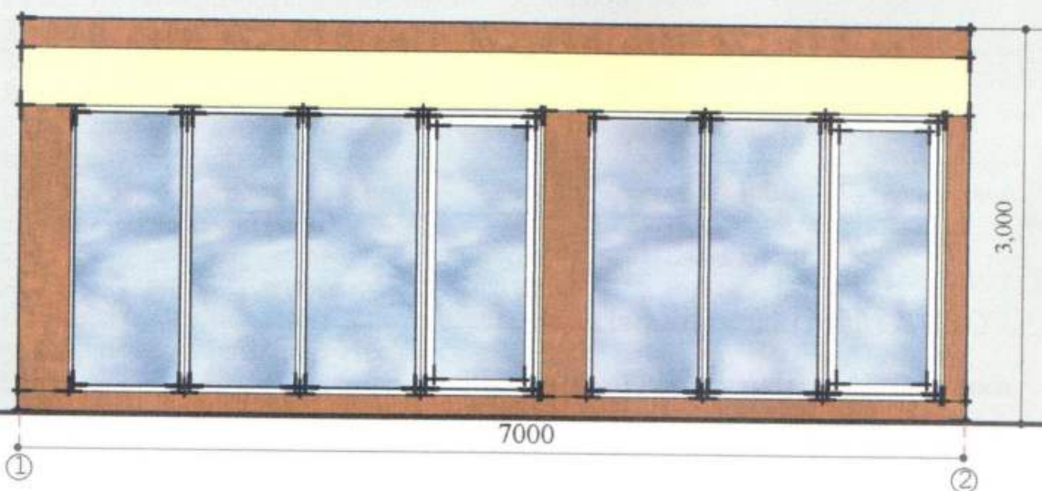
Боковий фасад
