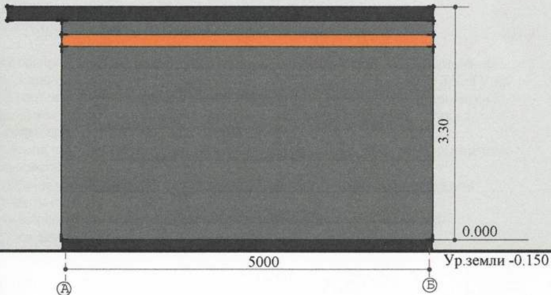
Боковий фасад
