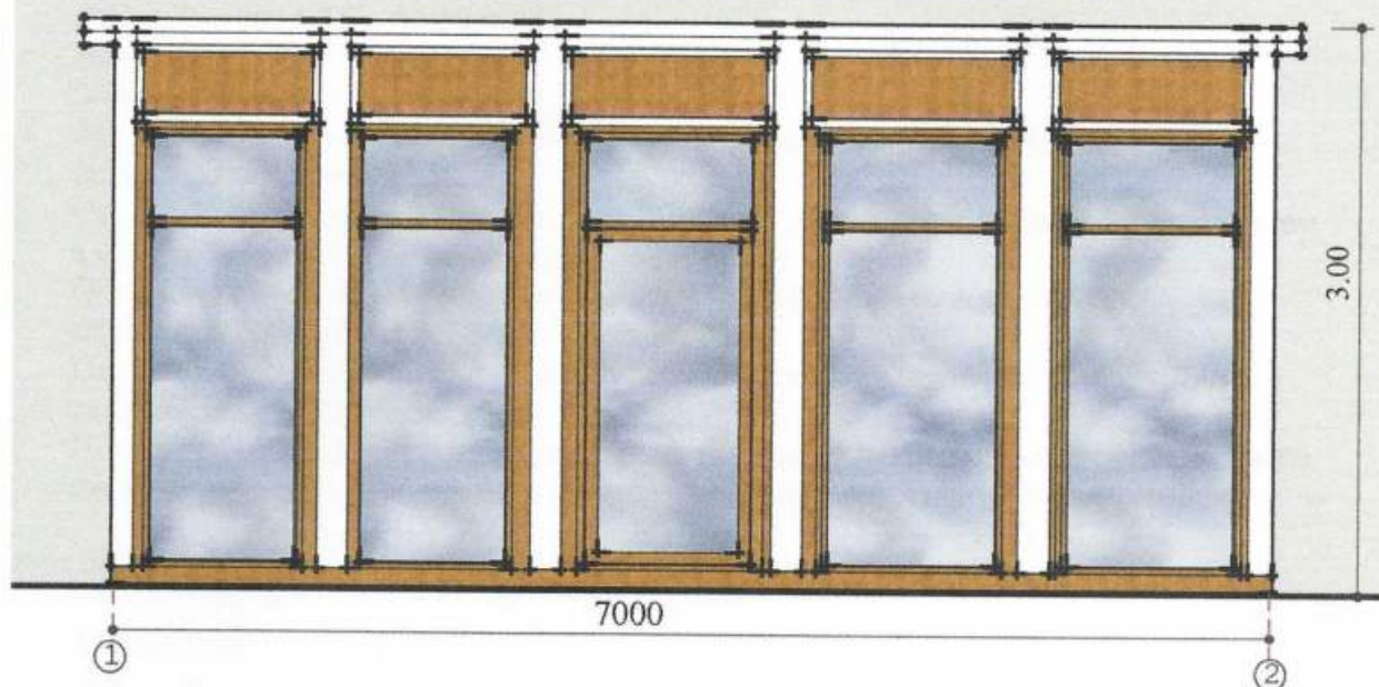
Боковий фасад
