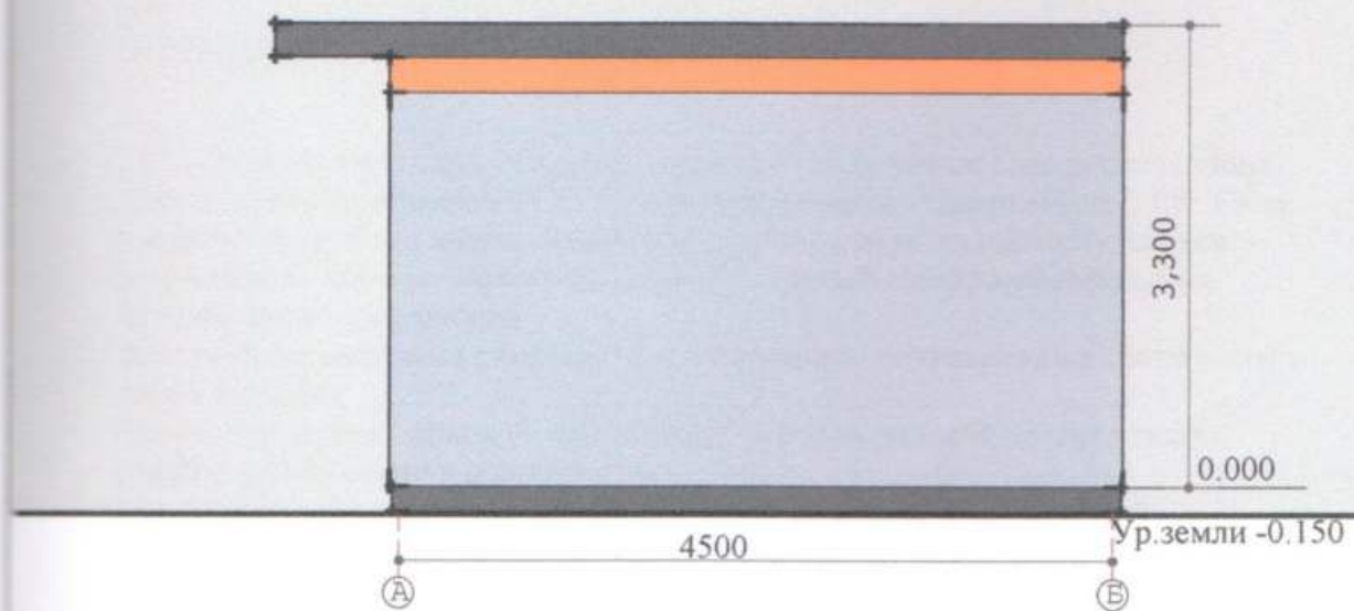
Боковий фасад
