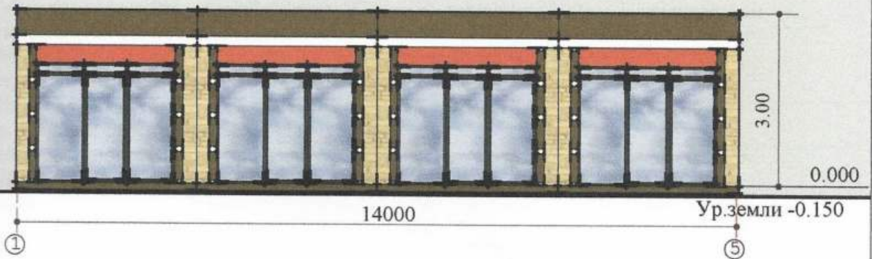
Боковий фасад
