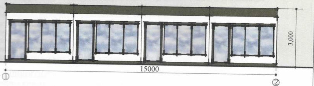
Боковий фасад м. 1:50
