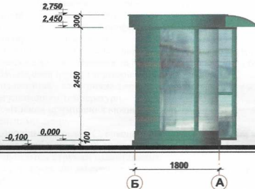
Бічний фасад
