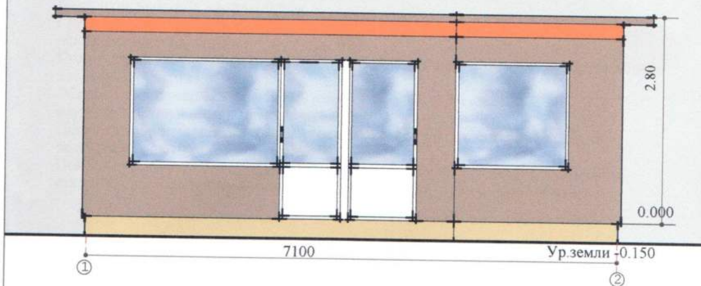
Боковий фасад
