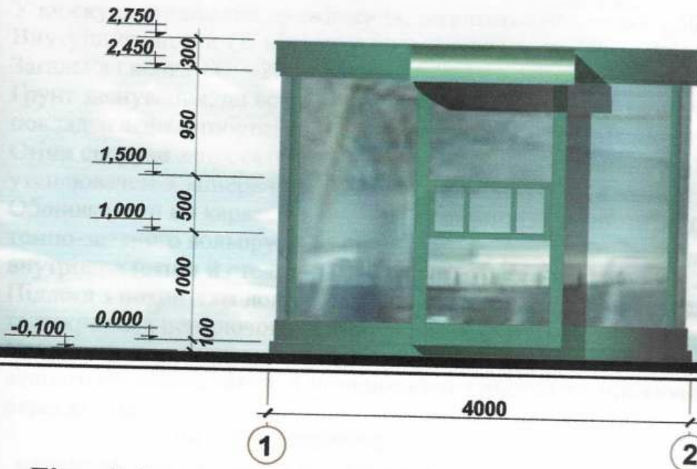
Бічний фасад
