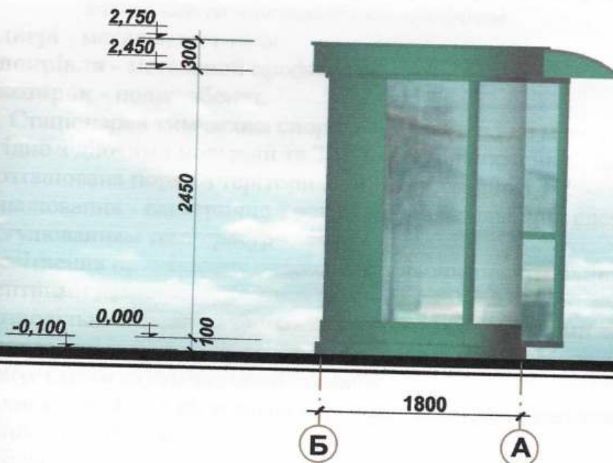
Бічний фасад
