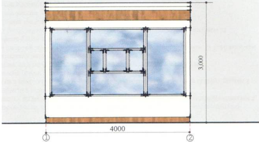
Боковий фасад
