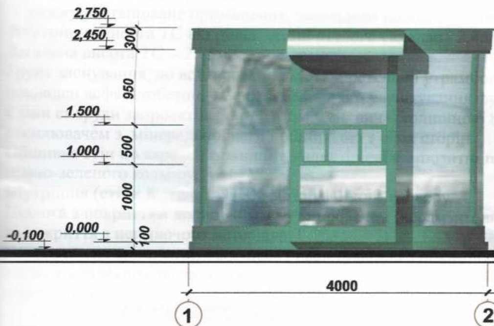
Бічний фасад
