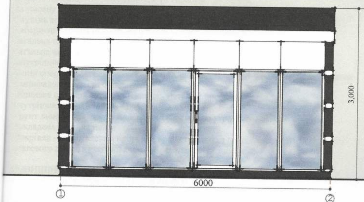
Боковий фасад
