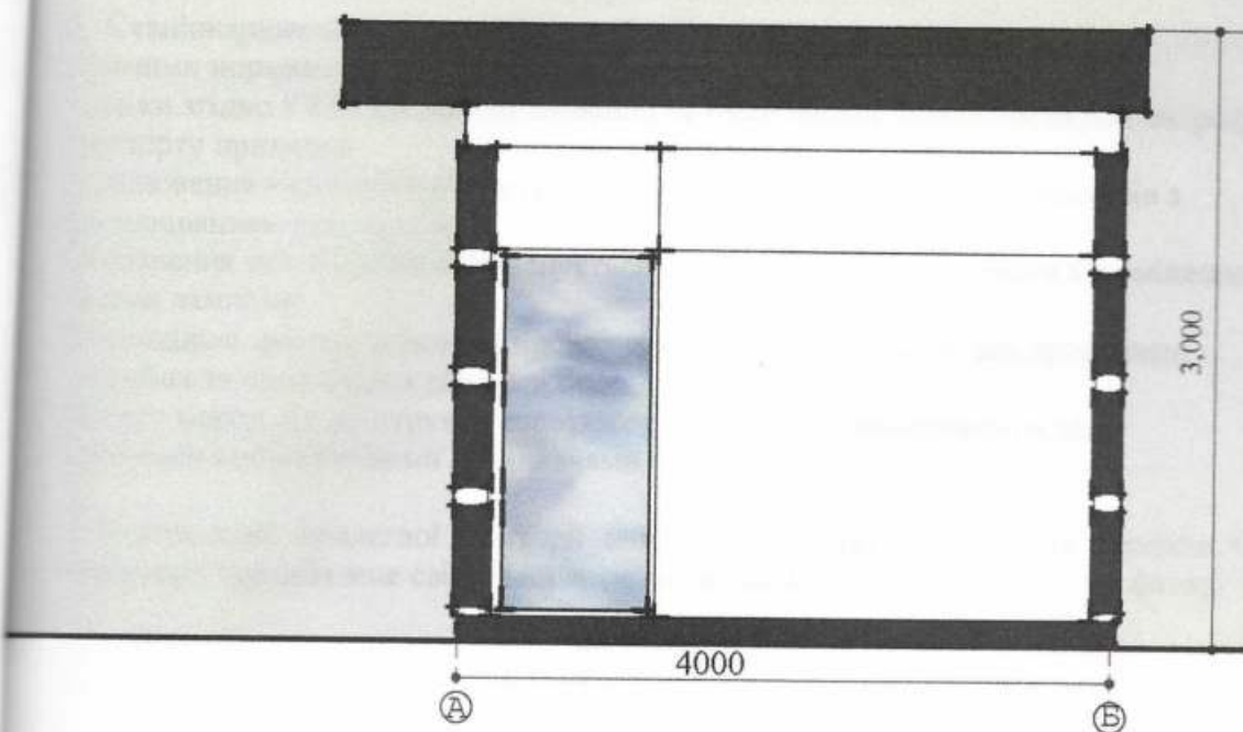
Боковий фасад
