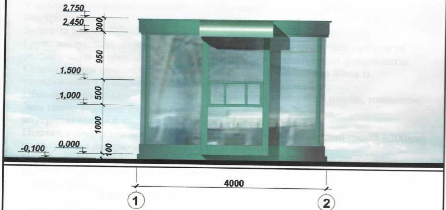
Бічний фасад
