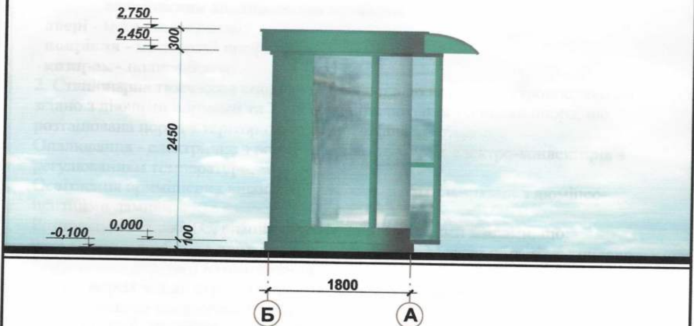
Бічний фасад
