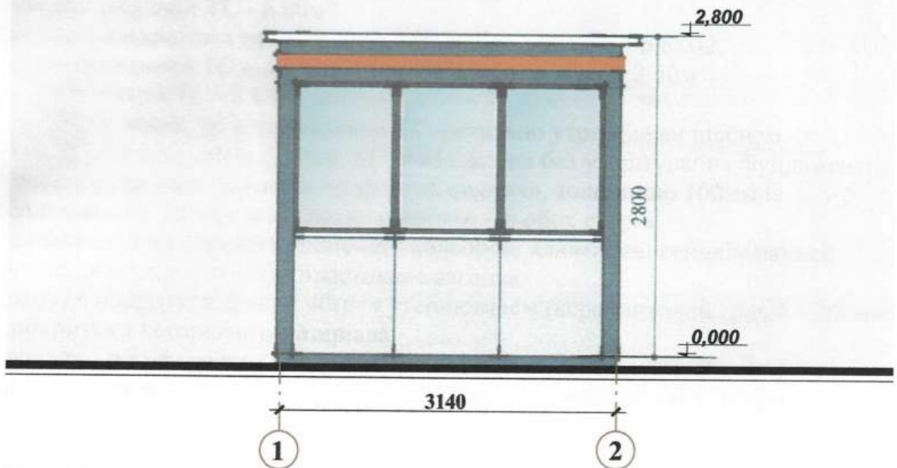
Бічний фасад
