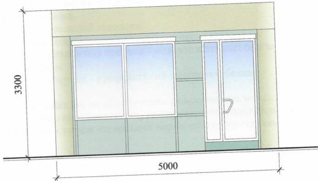
Головний фасад ТС М 1:50
