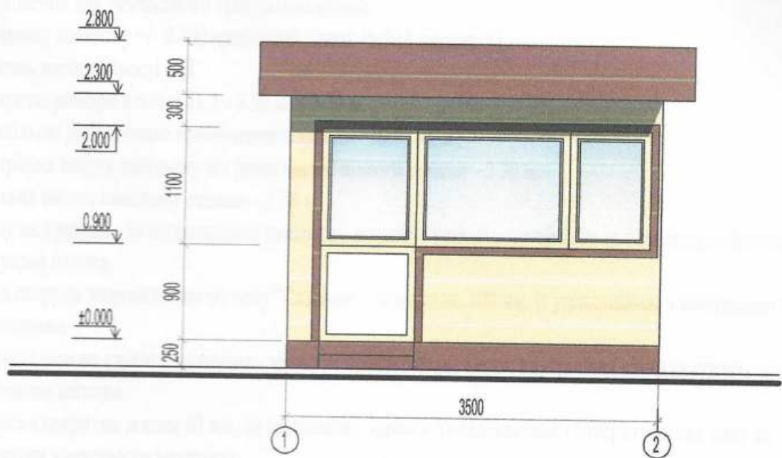
Фасад в осях "1"- "2", М 1:50
